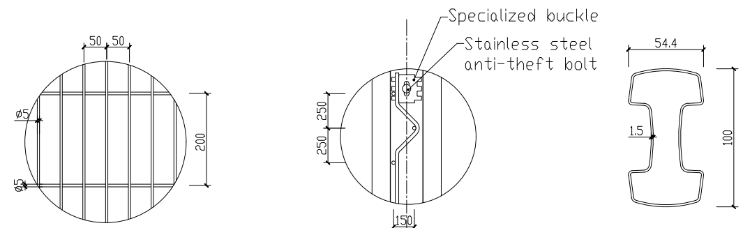
Node B 4:1
